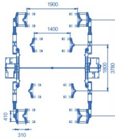
זרועות לליפט שני עמודים 5.5 טון OMCN 199/WRX
